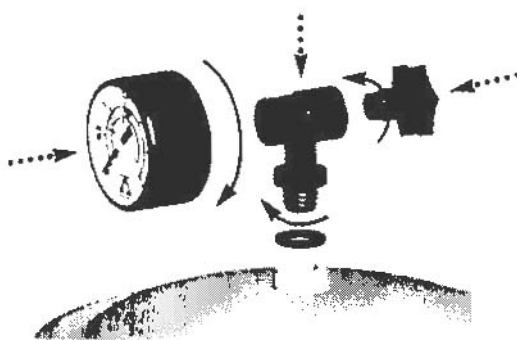
Montaje manómetro válvula lateral
