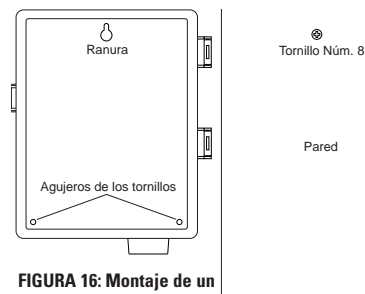
FIGURA 16: Montaje de un programador de interior
